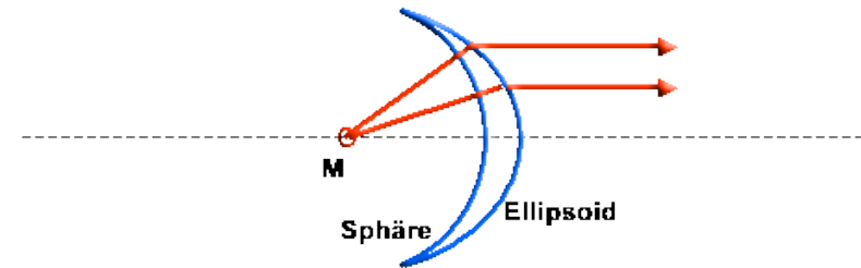
Bild 5.7: Sphäroelliptische Konvexlinse
