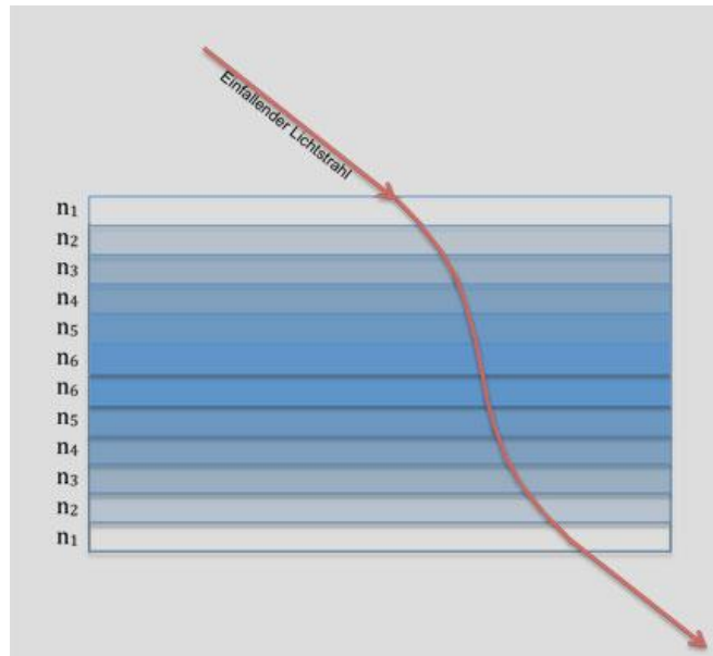
Bild 11.5: Ein Lichtstrahl durchläuft einen Glasplattenstapel mit gestaffeltem Brechungsindex.
