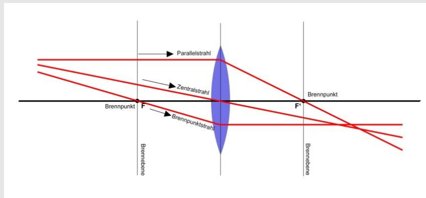
Bild 7.4 Strahlverläufe an dünnen Linsen – Parallel-, Zentral-, Brennpunktstrahl
