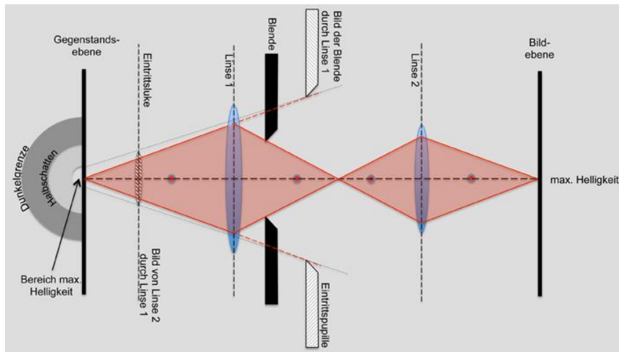
Bild 10.20: Bereich maximaler Helligkeit.
