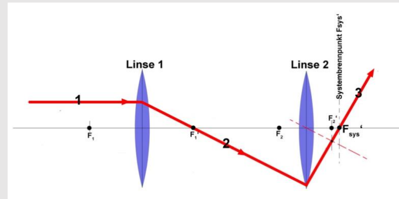
Bild 8.10: Konstruktion des Systembrennpunktes F_{\text{sys}}' auf der Bildseite.
