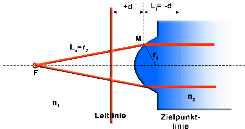
Bild 5.5: Strahlverlauf durch eine hyperboloidförmige brechende Fläche. (Der Abstand der Leitlinie von dem Punkt M auf der Oberfläche ist +d . L_i = -d ist der Abstand der Zielpunkte innerhalb des Hyperboloids.)
