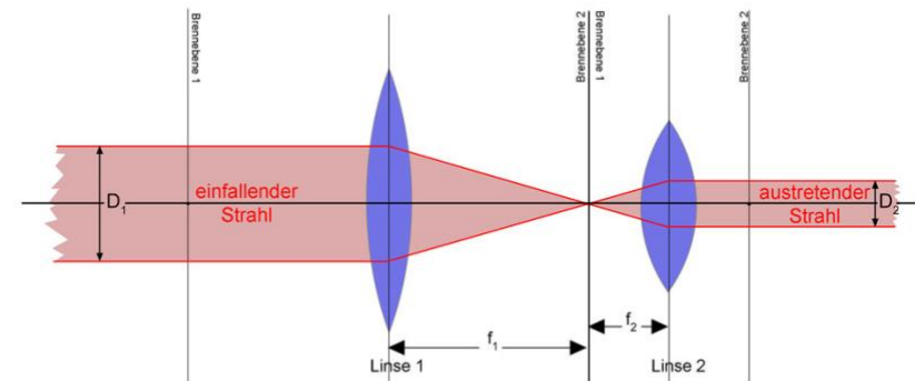
Bild 8.19 Teleskopischer Strahlengang (Reduzierung des Strahldurchmessers.)
