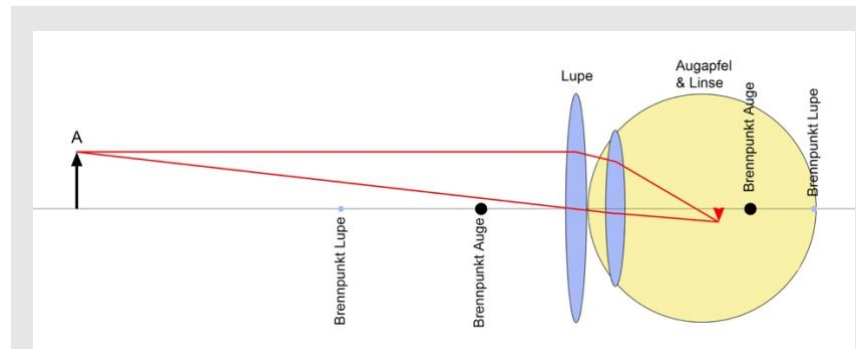
Bild 9.13: Abbildung durch eine Lupe, dicht vor dem Augapfel
