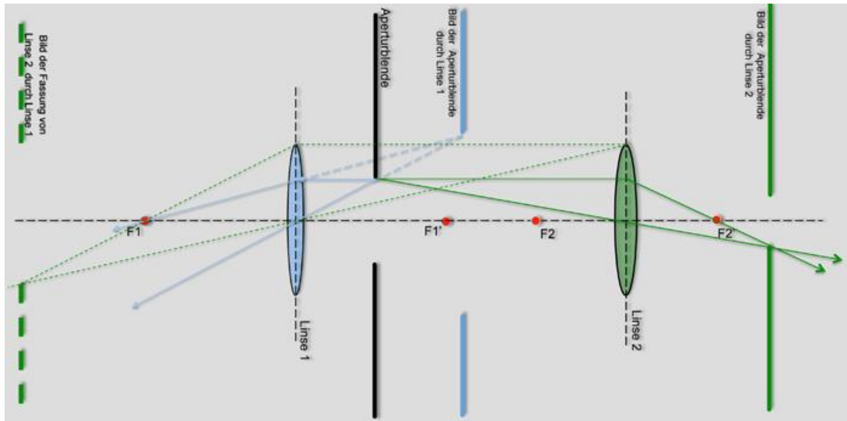
Bild 10.11: Konstruktion der Bilder der Aperturblende (Pupillen). Eine detaillierte Beschreibung wie man eine Abbildung durch eine dünne Linse konstruiert finden Sie im Kapitel 8.
