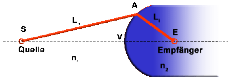
Bild 5.1: Prinzipbild zur Oberflächenform eines fokussierenden Elementes - Strahlverlauf durch eine asphärische Fläche.
