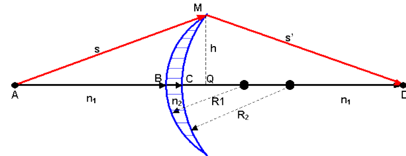
Bild 7.1: Kenndaten einer „dünnen“ Linse.
