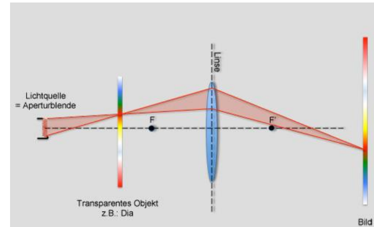
Bild 10.23: Lichtquelle (Lampenwendel) als Aperturblende.
