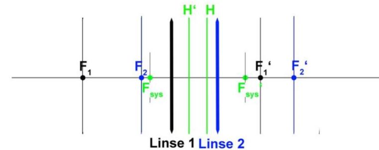
Bild 8.27: Linsensystem (Linse 1 und Linse 2) mit den zugehörigen Einzelbrennweiten ( F_1 , F_1' , F_2 , F_2' ) und den Hauptebenen H und H' .
