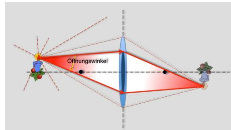
Bild 10.4: Apertur- oder Öffnungsblende.
