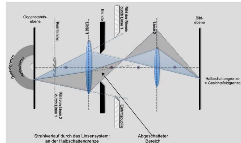
Bild 10.22: Halbschatten-, Gesichtsfeldgrenze
