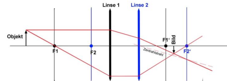
Bild 8.29: Abbildungsstrahlengang durch das Linsensystem aus Bild 8.27
