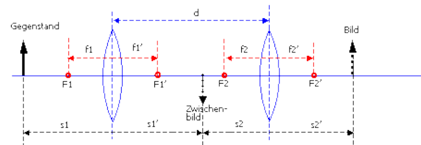
Bild 8.9: 2-Linsensystem
