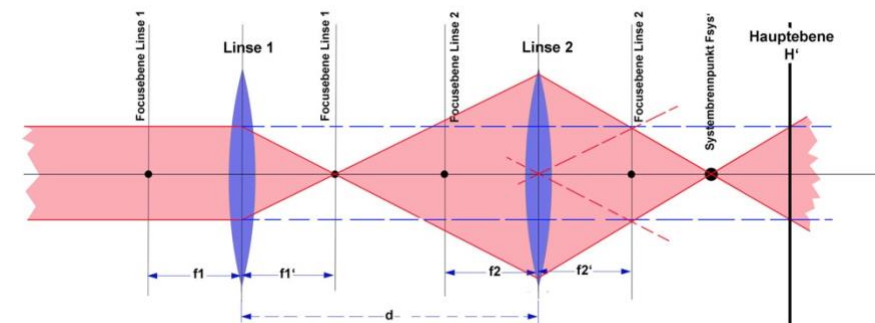
Bild 8.23: Hauptebene eines Linsensystems aus zwei „dünnen“ Bikonvexlinsen.
