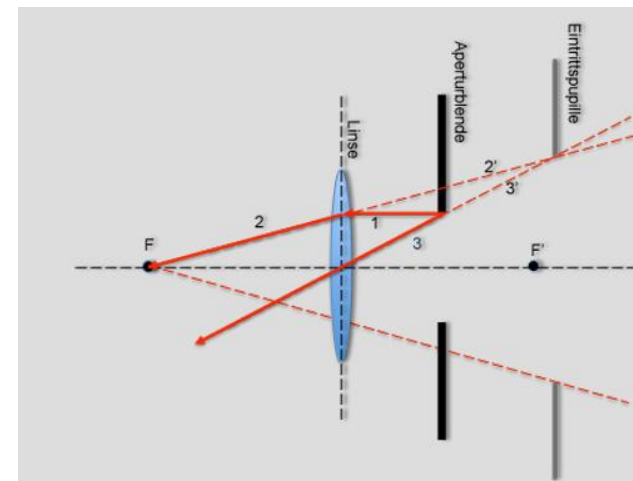
Bild 10.7: Konstruktion der Eintrittspupille.
