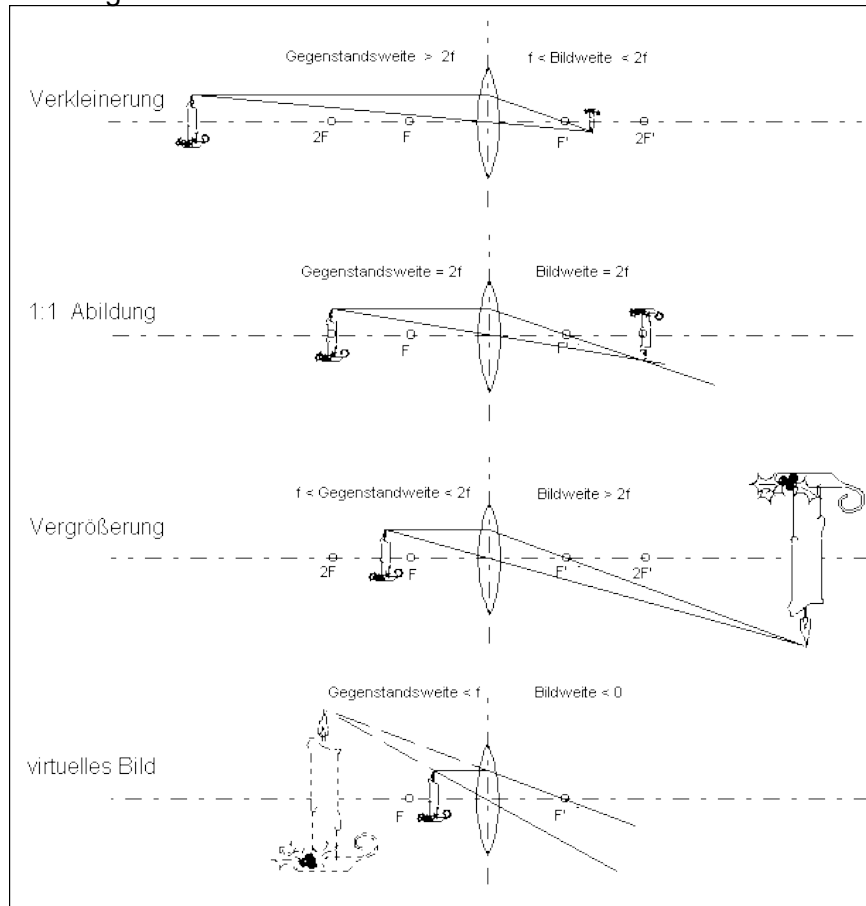
Bild 8.3: Abbildung durch eine dünne Linse bei verschiedenen Gegenstandsweiten.
