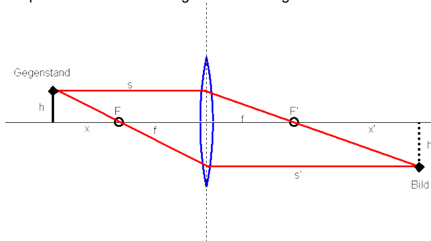
Bild 8.2: Abbildung durch eine dünne Linse.
