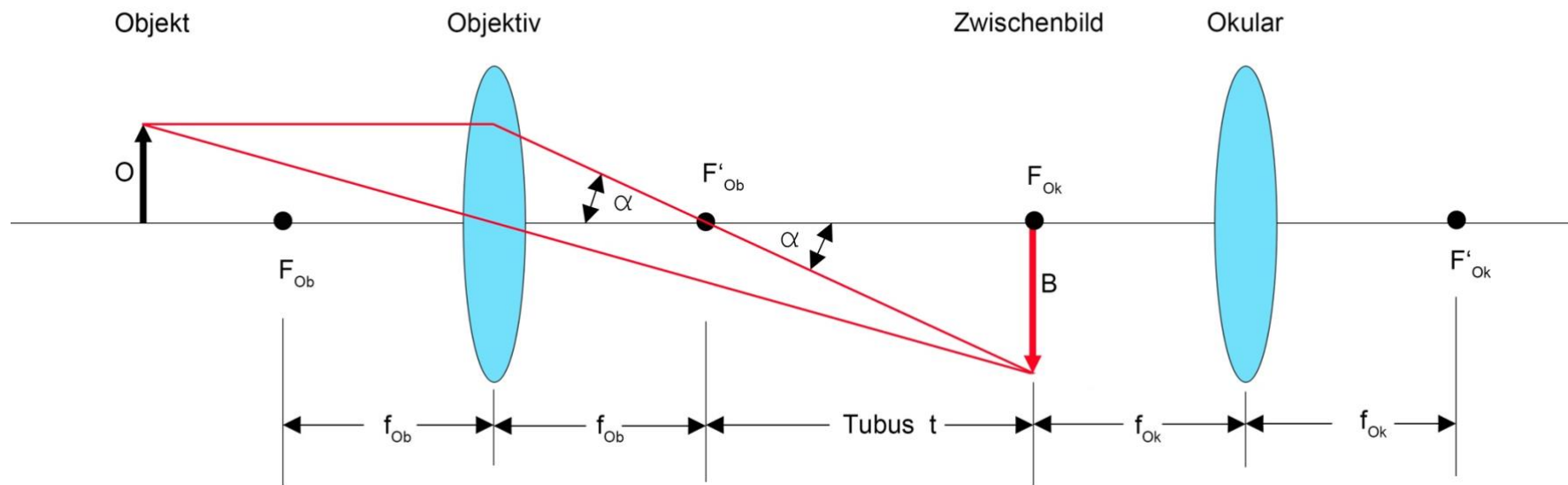
Bild 9.22: Abbildungsstrahlengang durch ein Mikroskopobjektiv.
