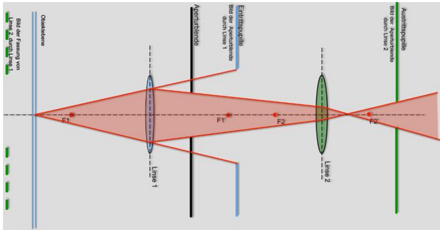
Bild 10.14: Strahlenkegel durch ein Linsen- / Blendensystem: konstruiert mit Hilfe von Blenden und Pupillen
