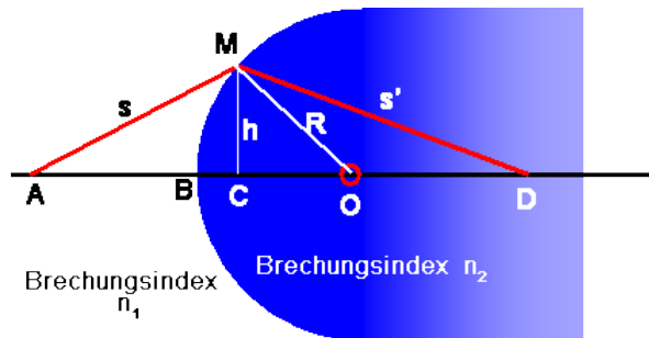
Bild 6.3: Brechung an einer kugelförmigen Grenzfläche. (Kenngrößen)
