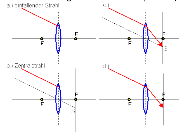
Bild 8.7: Konstruktion des Strahlverlaufes durch eine dünne Linse für einen beliebigen, schräg einfallenden Strahl.
