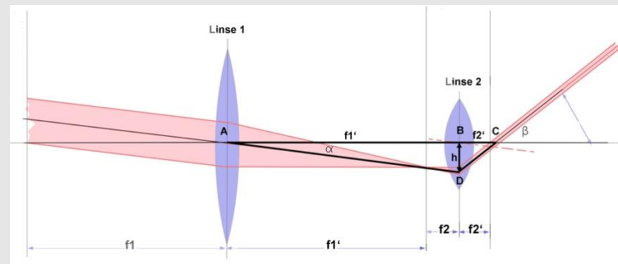
Bild 8.21: Konstruktionselemente eines teleskopischen Strahlengangs.
