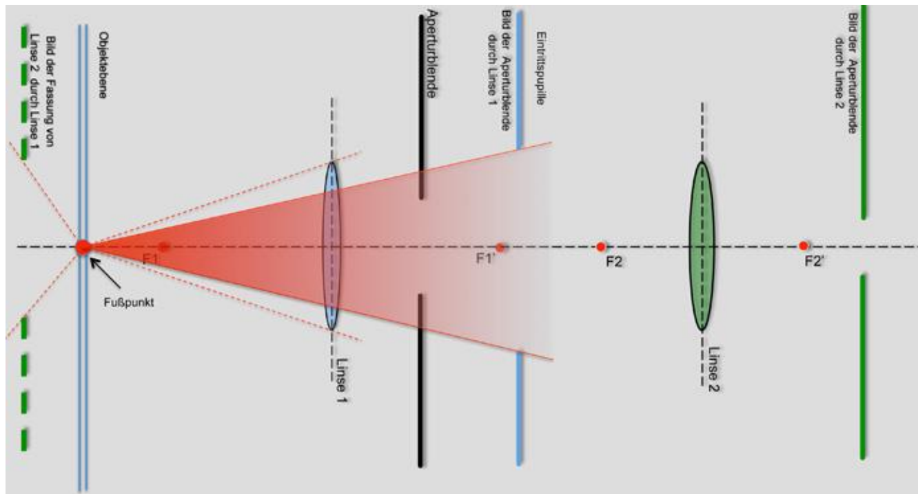
Bild 10.13: Bestimmung der Eintrittspupille.
