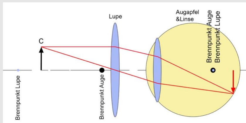
Bild 9.16: Abbildung durch eine Lupe in etwas größerem Abstand von Augapfel.
