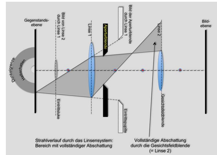
Bild 10.21: Dunkelgrenze
