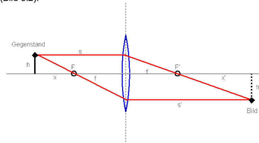
Bild 8.2: Abbildungsstrahlengang durch eine „dünne“ Linse.
