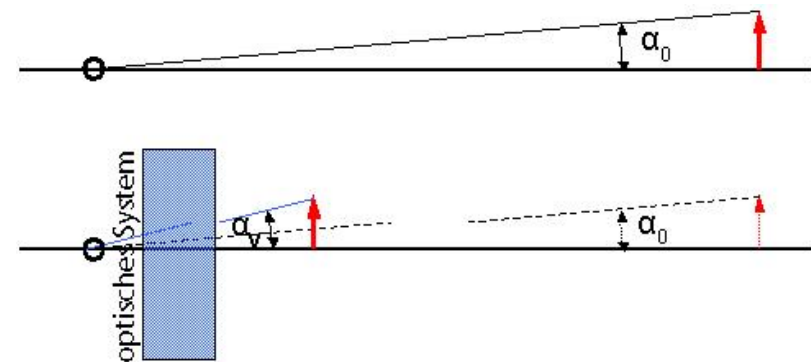
Bild 9.1: Winkelvergrößerung
