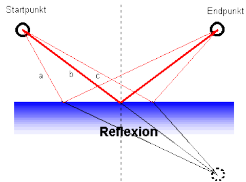
Bild 2.3: Reflexion – auf der Suche nach dem kürzesten Weg.
