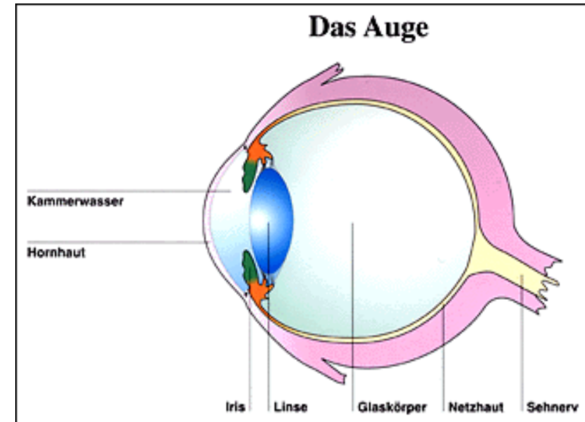
Bild 9.2: Das Auge
