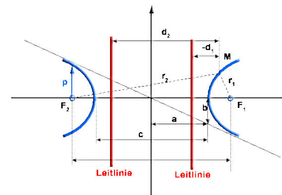
Bild 5.4: Kenngrößen der Hyperbel.
