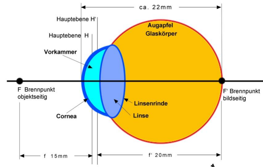
Bild 9.3: Die wichtigsten (optischen) Elemente im Auge.
