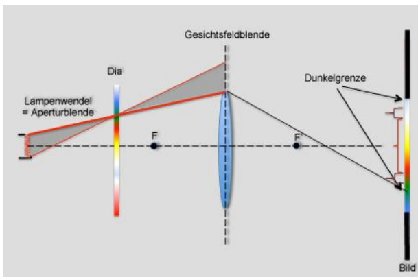
Bild 10.28: Bestimmung der Dunkelgrenze.
