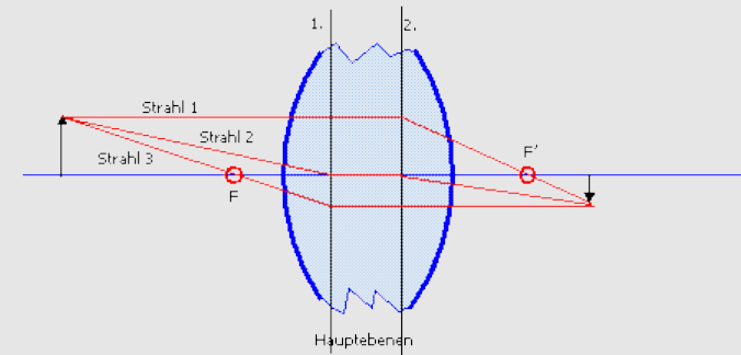
Bild 8.22. „Dicke“ Linse mit Hauptebenen.
