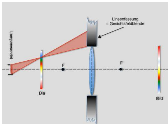
Bild 10.25: Linsefassung als Gesichtsfeldblende.
