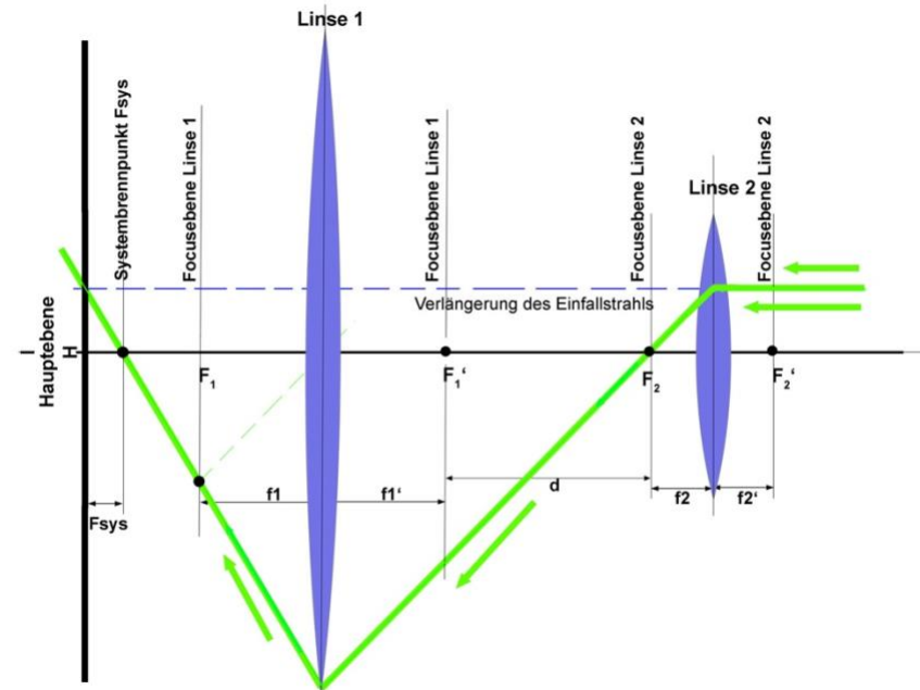
Bild 8.25: Konstruktion der objektseitigen Hauptebene H und des Systembrennpunktes F_{\text{sys}} für einen von rechts (Bildseite) einfallenden Strahl.
