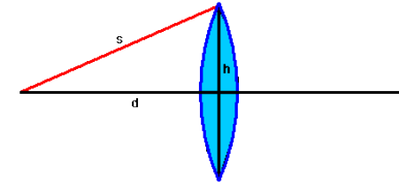
Bild 6.2 Kenngrößen für die Geometrie einer Linse mit kugelförmigen Grenzflächen.
