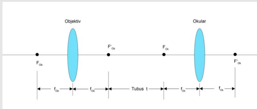
Bild 9.21: Grundkomponenten eines Mikroskops: Objektiv und Okular.
