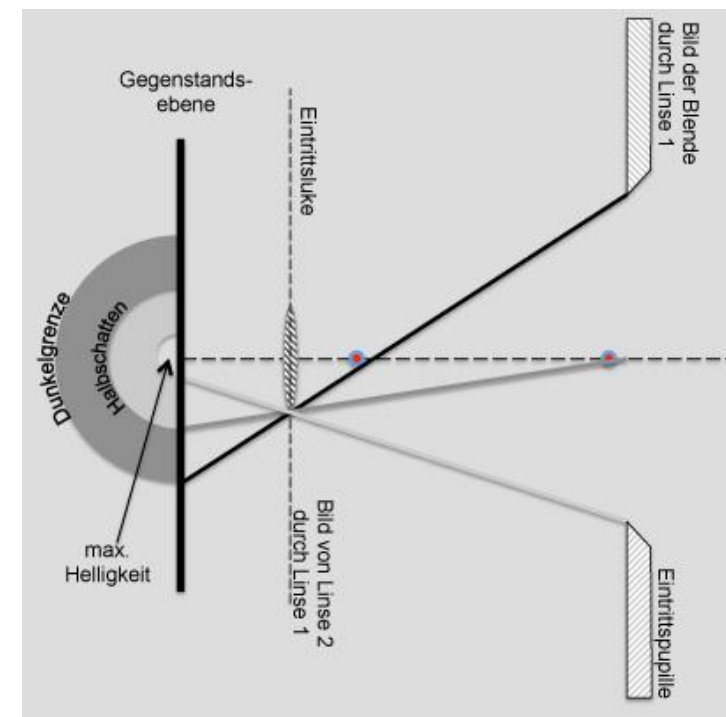
Bild 10.19: Bestimmung des Gesichtsfeldes.
