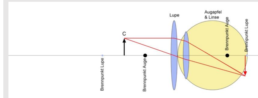
Bild 9.14: Abbildung durch eine Lupe, dicht vor dem Augapfel
