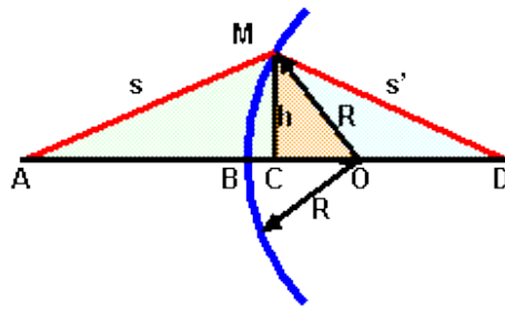
Bild 6.4: Beziehung für die Schnittweiten s und s' bei einer kugelförmigen Grenzfläche.
