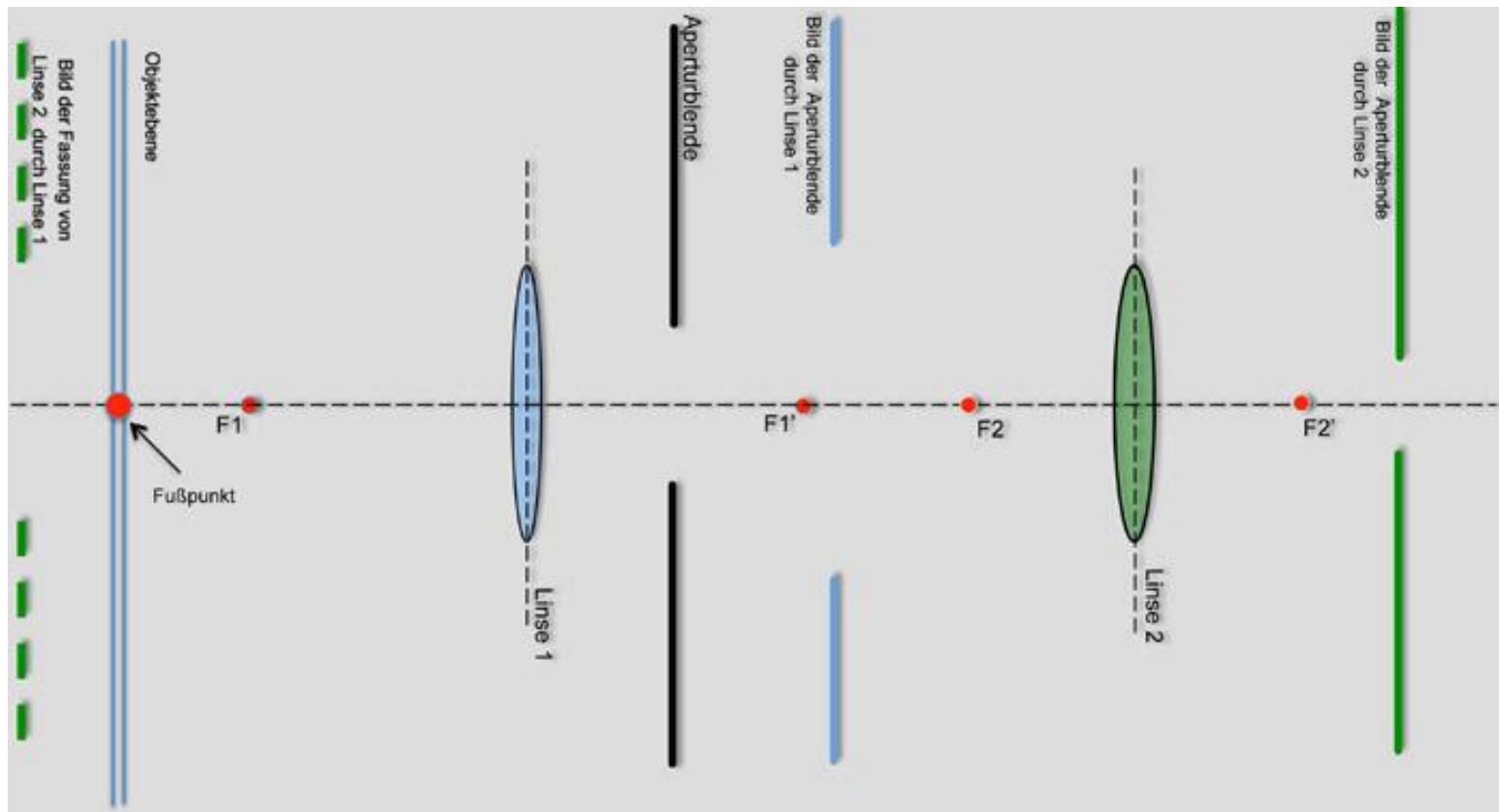
Bild 10.12: Linsensystem mit sämtlichen Bildern der Aperturblende (Pupillen)
