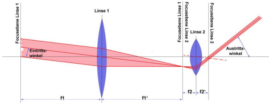
Bild 8.20 Teleskopischer Strahlengang – (Winkelvergrößerung)
