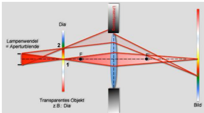
Bild 10.24: Vignettierung im Beleuchtungsstrahlengang.
