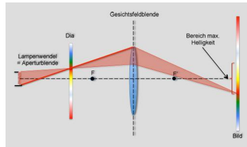
Bild 10.26: Bereiche maximaler Helligkeit.
