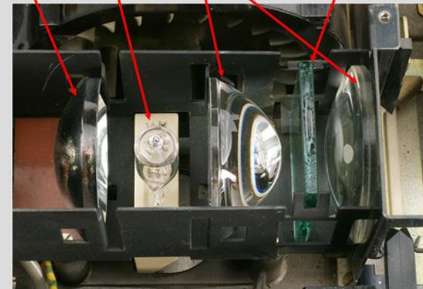
Bild 10.31: Das Lampengehäuse eines Dia-Projektors.
