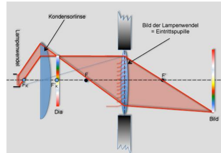
Bild 10.30: Abbildungsstrahlengang mit Kondensorlinse in einem (Dia-)Projektor.
