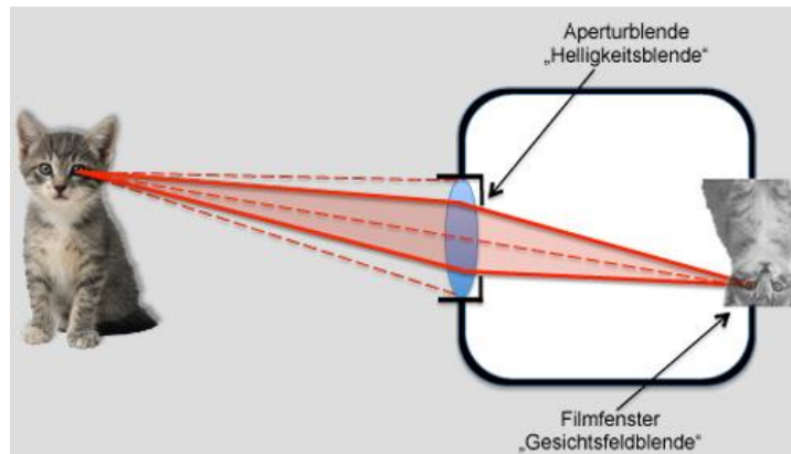
Bild 10.5: Prinzipskizze eines einfachen Fotoapparates mit Aperturblende.
