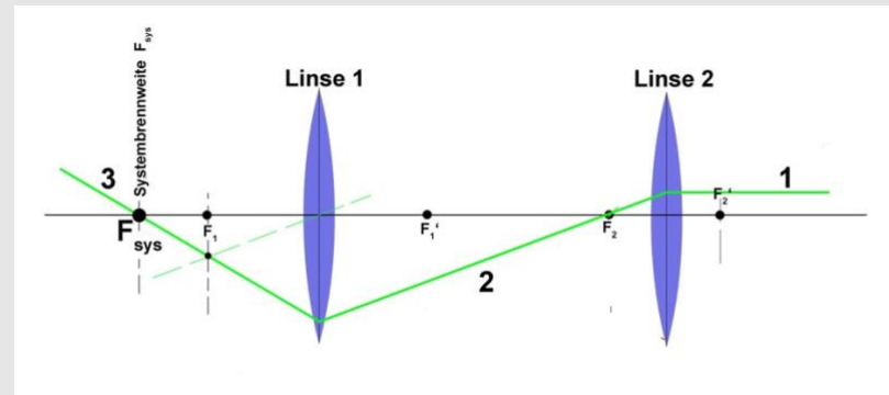
Bild 8.11: Konstruktion des Systembrennpunktes F_{\text{sys}} auf der Gegenstandsseite. (Konstruktion des Strahlverlaufes – analog zu Bild 8.10)
