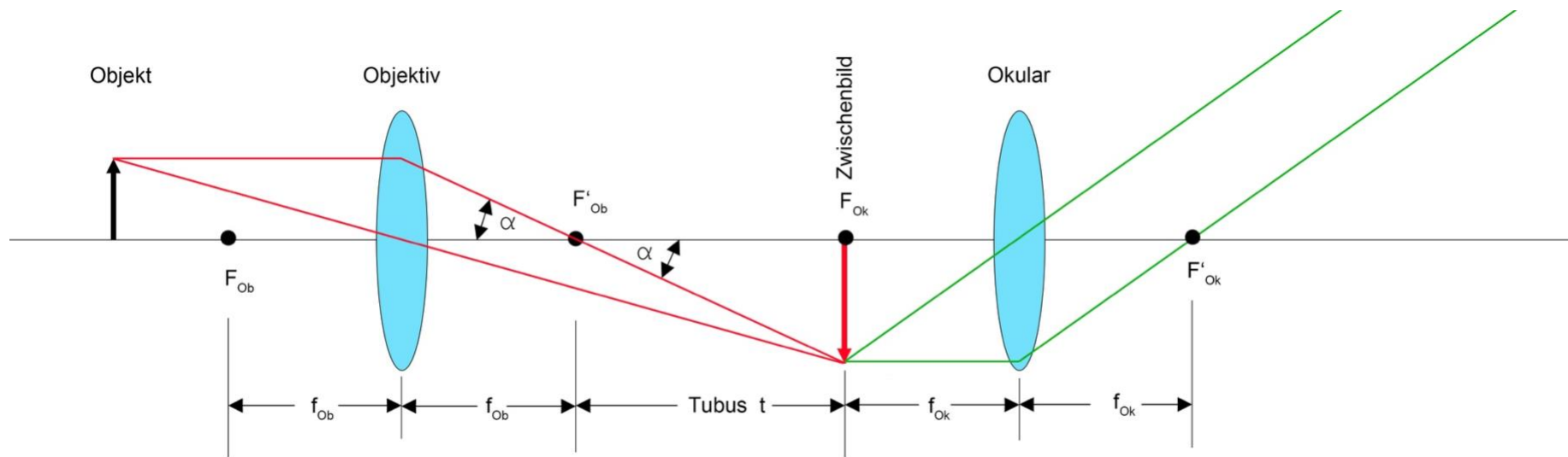
Bild 9.24 Mikroskopstrahlengang – Zwischenbild im Okularbrennpunkt
