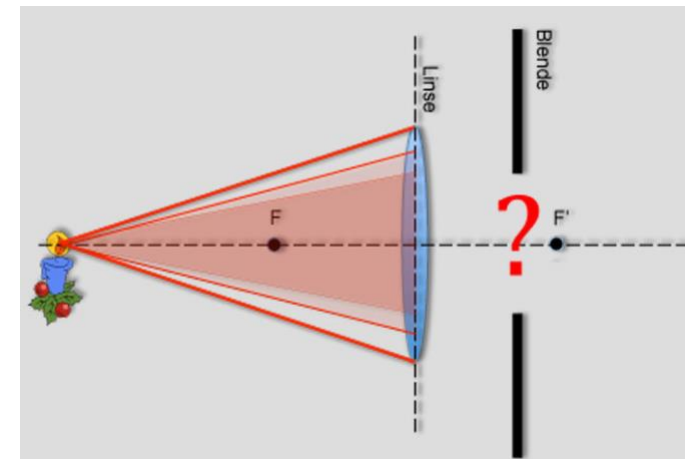
Bild 10.3: Blende hinter einer Linse. Wie wirkt sich das auf die Bildhelligkeit aus?
