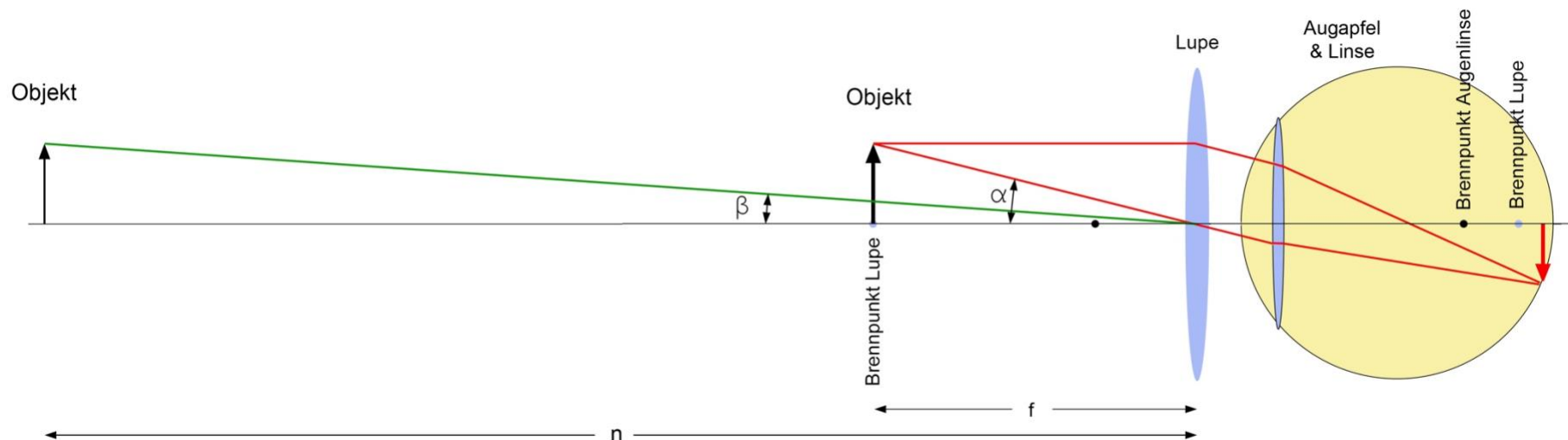
Bild 9.17 Prinzipbild zur Definition der Winkelvergrößerung bei der Lupe:
