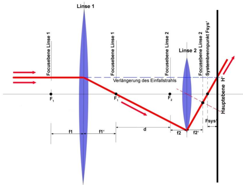
Bild 8.24: Konstruktion der bildseitigen Hauptebene H' und des Systembrennpunktes F_{sys}' für einen von Links (Objektseite) einfallenden Strahl.
