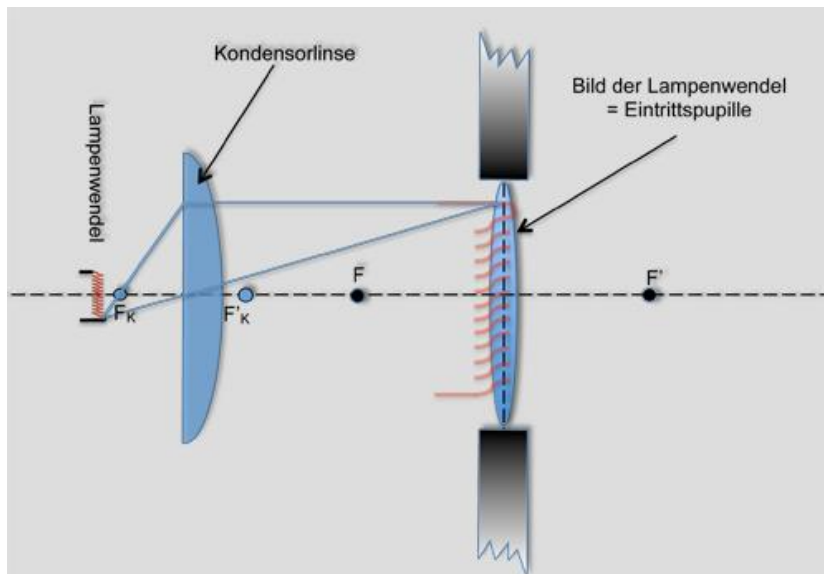
Bild 10.29: Wirkung einer Kondensorlinse im Abbildungsstrahlengang eines Diaprojektors.
