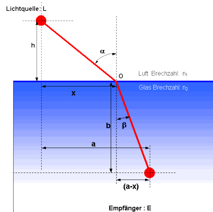
Bild 3.3: Parameter zur Brechung.
