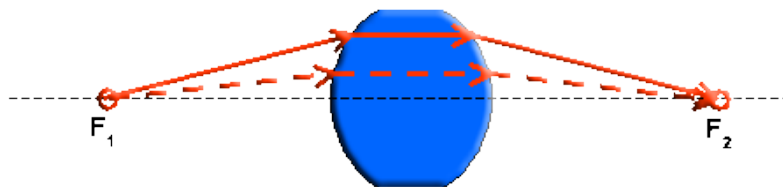
Bild 5.6: Hyperbolische Bikonvexlinse
