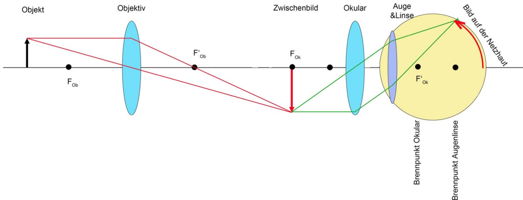
Bild 9.25: Versuch der Darstellung eines vollständigen Mikroskopstrahlenganges
