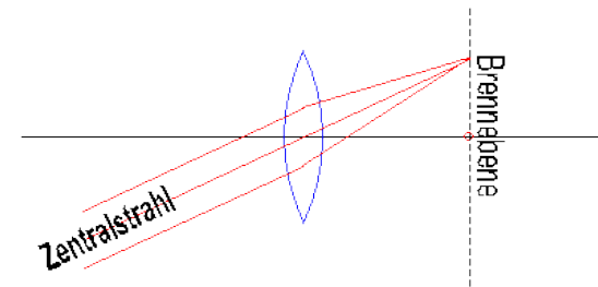
Bild 8.6: Schräg einfallendes Strahlenbündel wird in der Brennebene fokussiert
