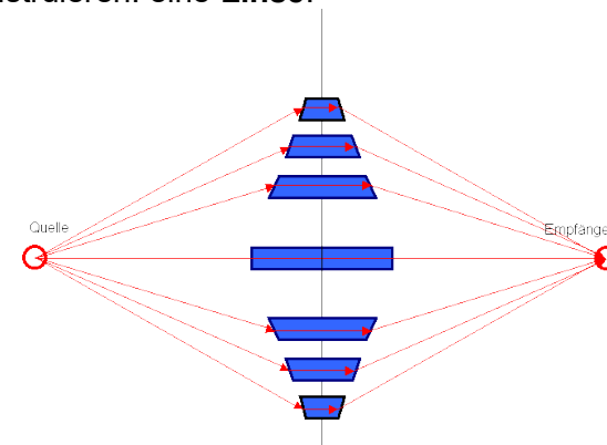
Bild 4.2: Prinzipbild zur Konstruktion eines fokussierenden Elementes.
