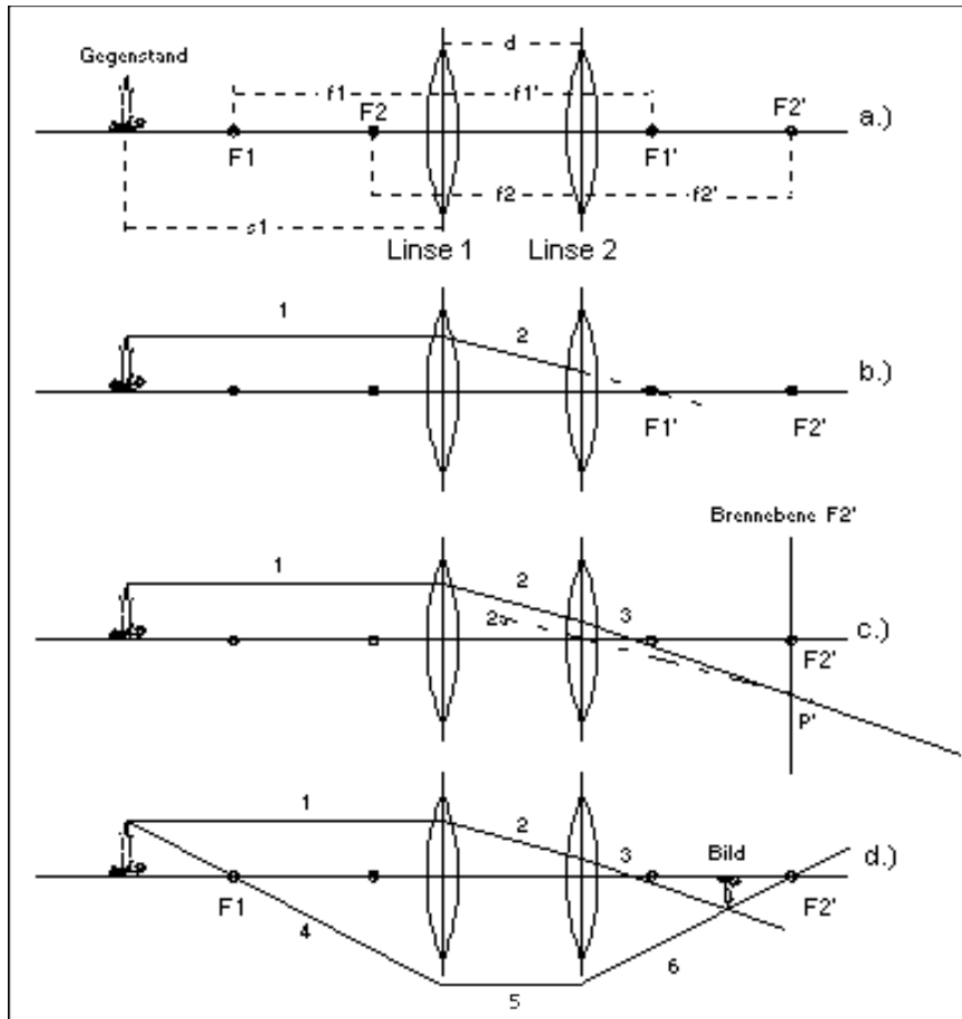
Bild 8.8: Abbildung durch ein Linsensystem
