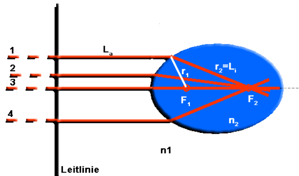
Bild 5.2: Brennpunkte ( F_1 u. F_2 ) einer ellipsoidförmigen Fläche ( n_1 < n_2 ).
