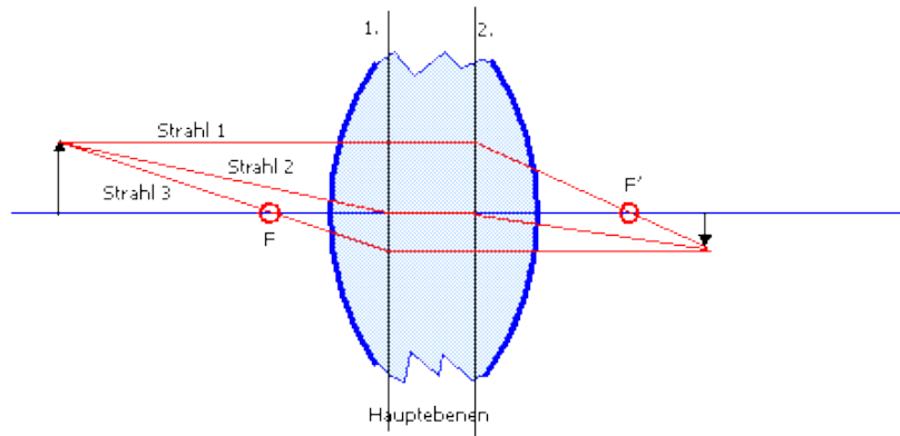
Bild 8.22: „Dicke“ Linse mit Hauptebenen
