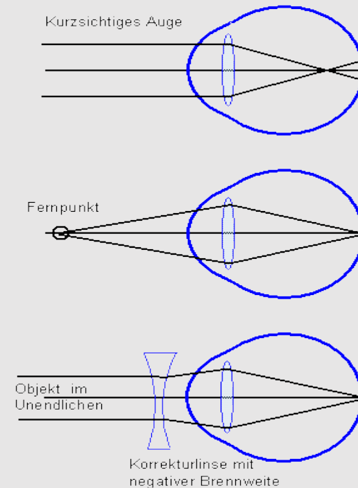
Bild 9.6: Kurzsichtiges Auge; Fernpunkt; Korrekturlinse mit negativer Brennweite.
