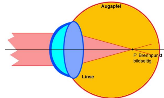
Bild 9.5: Kurzsichtigkeit
