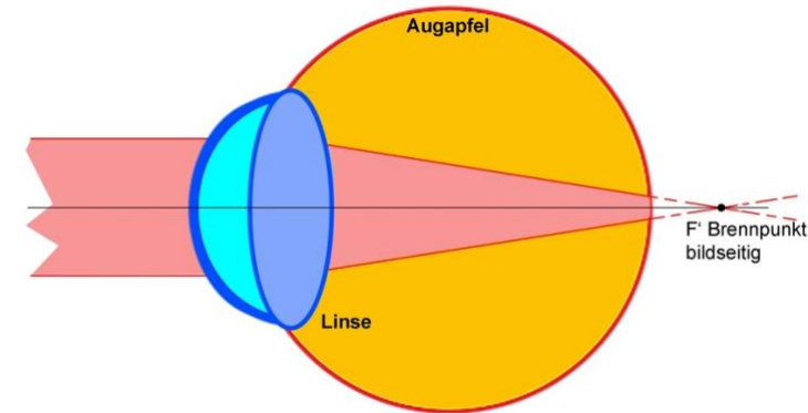
Bild 9.7: Weitsichtigkeit
