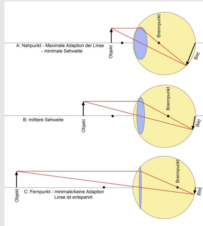
Bild 9.12: Objekt (schwarzer Pfeil) in unterschiedlichen Abständen vom Auge. Je näher das Objekt an das Auge herangeführt wird, um so mehr muss die Brennweite der Augenlinse durch den Ziliarmuskel verkürzt werden, damit eine scharfe Abbildung auf der Netzhaut entsteht.
