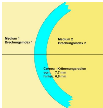
Bild 9.4: Prinzipbild der Cornea.
