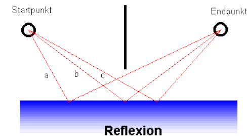
Bild 2.2: Reflexion – welches ist der kürzeste Weg?
