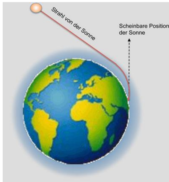
Bild 11.3: Verlauf eines Lichtstrahls in der Erdatmosphäre.
