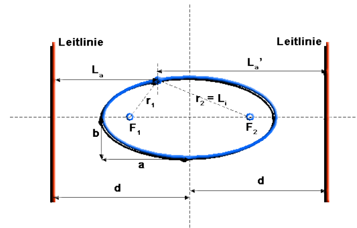
Bild 5.3: Kenngrößen der Ellipse.
