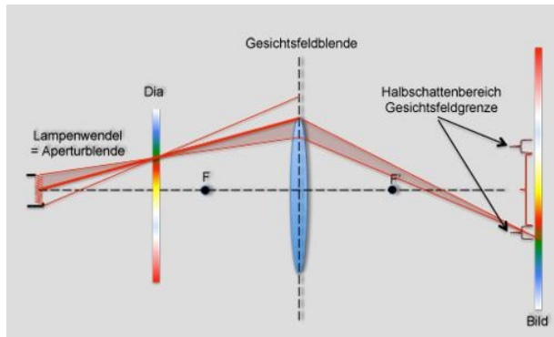
Bild 10.27: Bestimmung der Gesichtsfeldgrenze.
