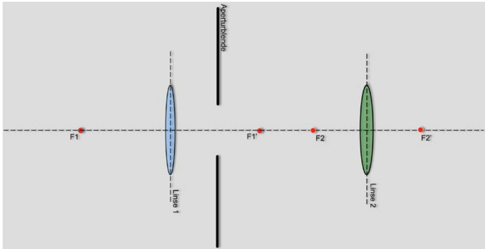
Bild 10.10: Beispielsystem (zwei Linsen und eine Blende) zur Konstruktion der Pupillen.
